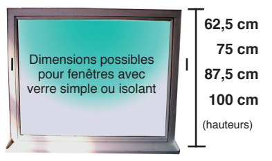
75 - 87,5 - 100 - 112,5 - 125 cm (largeurs)
