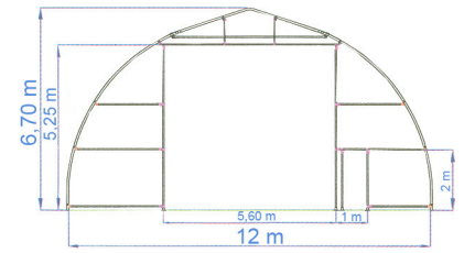
ARMATURE PIGNON AVEC PORTE
